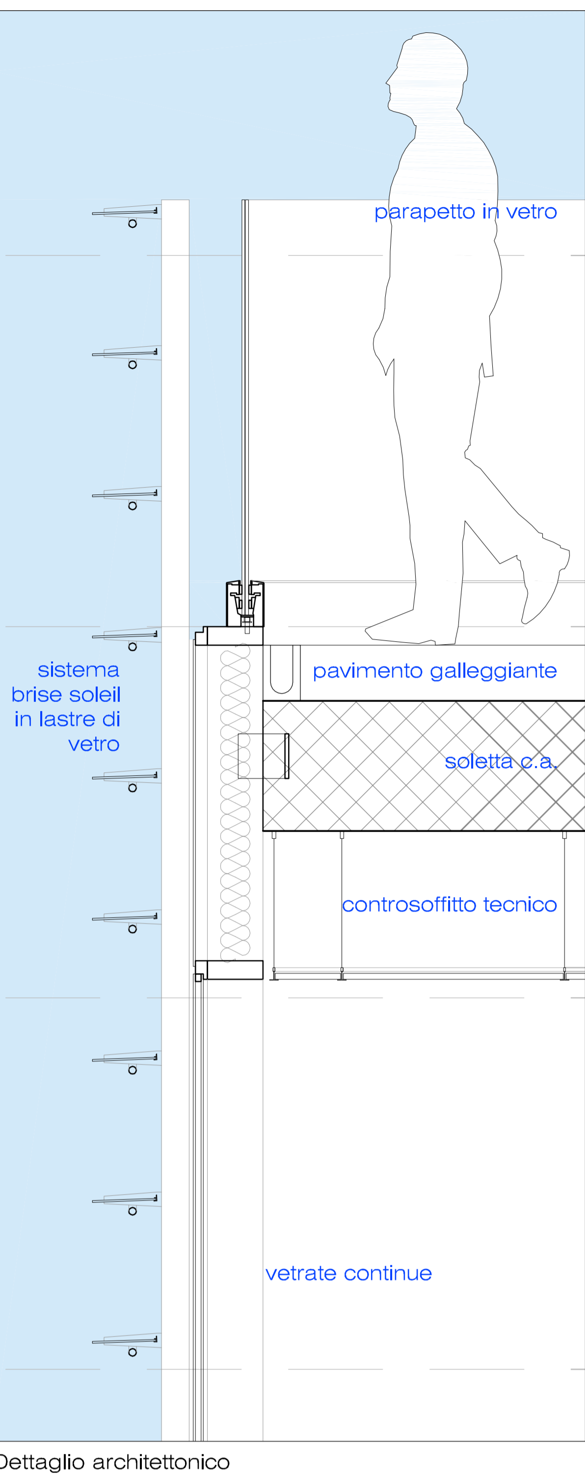
Dettaglio architettonico
