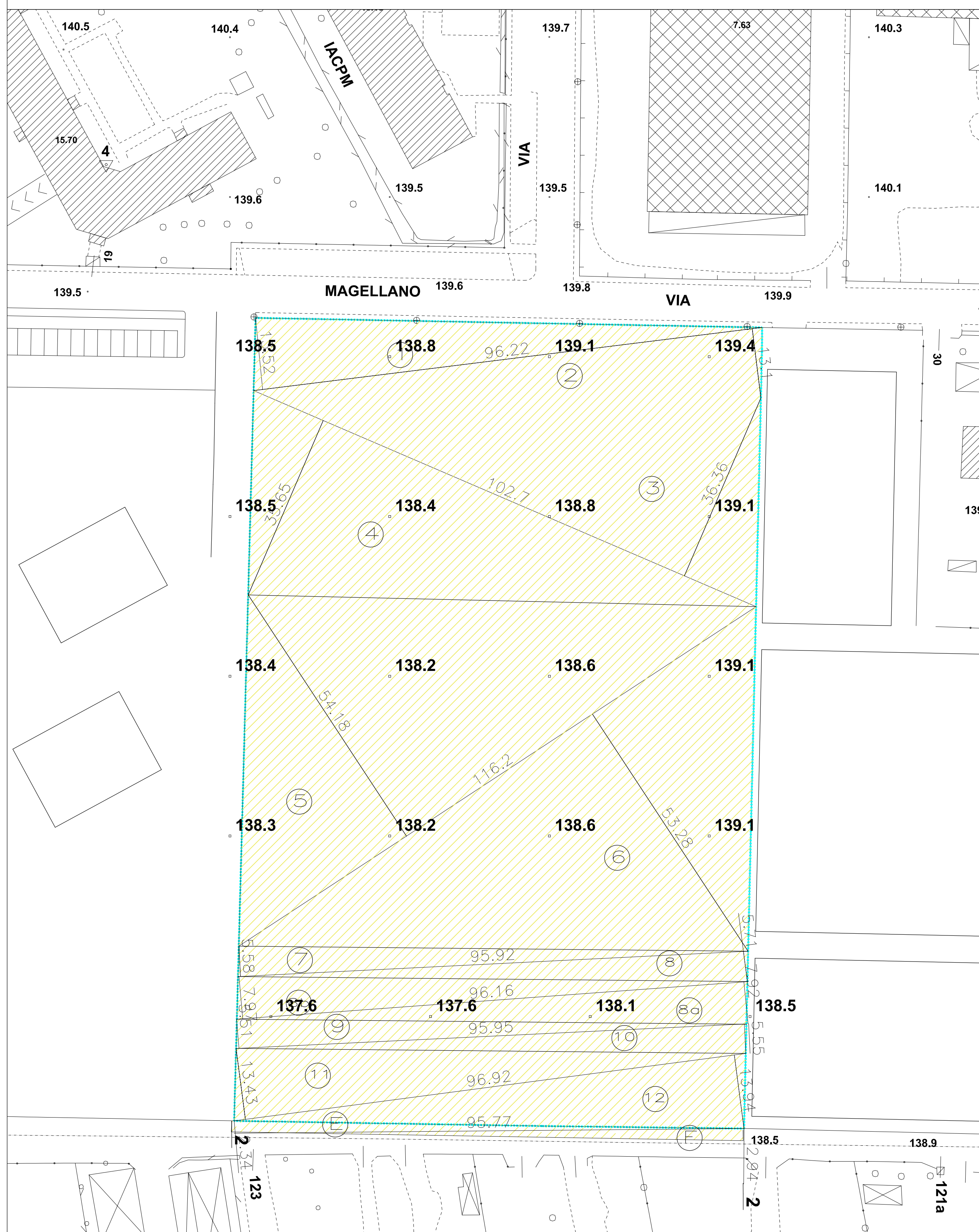
RILIEVO PROPRIETA' SCALA 1:500
